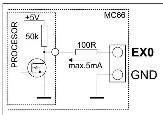
Schemat zastępczy układu wyjścia złącza EX0
