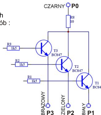
Schemat stopni wyjściowych przełącznika PS4
